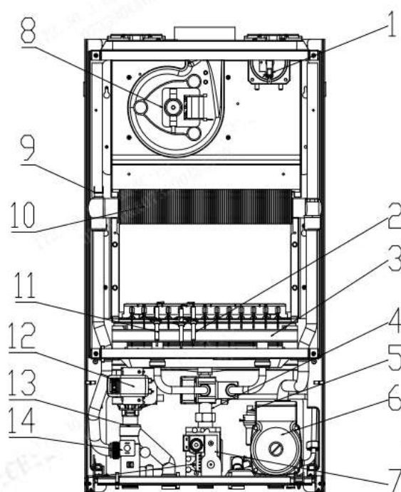
Одноконтурные
