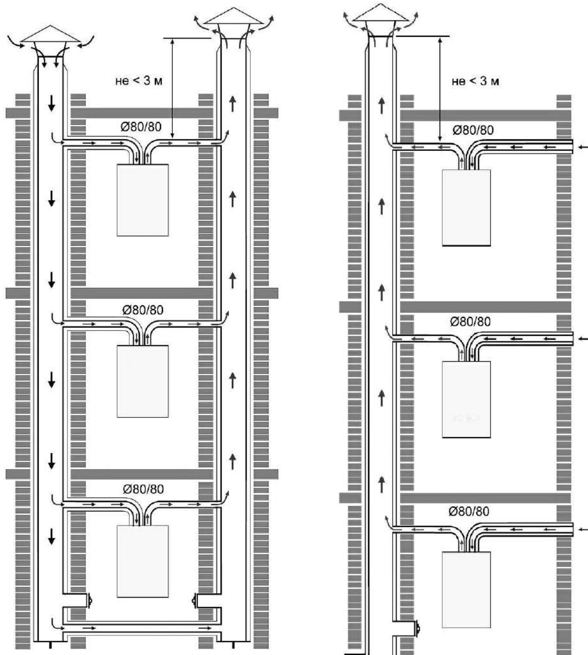
Схема установки раздельной системы дымоходов в многоквартирном доме
