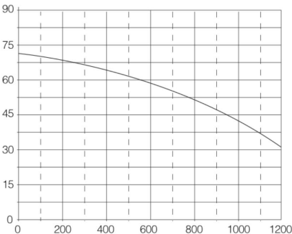
Расход (л/ч)
