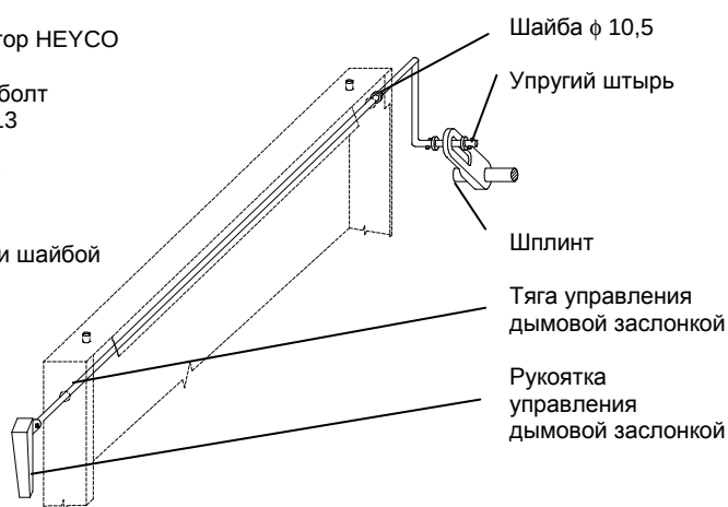
Рис. 12 Управление дымовой заслонкой
