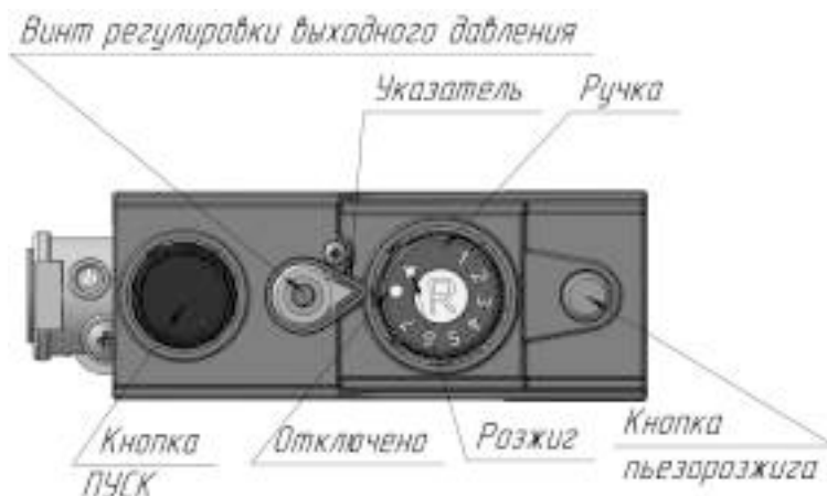
Рисунок 3. Элементы управления на газовом блоке автоматики САБК-АТ.
